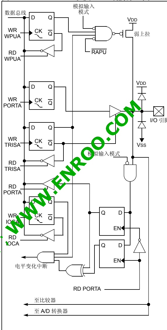
图 3-1: RA0 以及 RA1 引脚原理图
