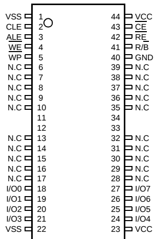
44(40) TSOP (II)
