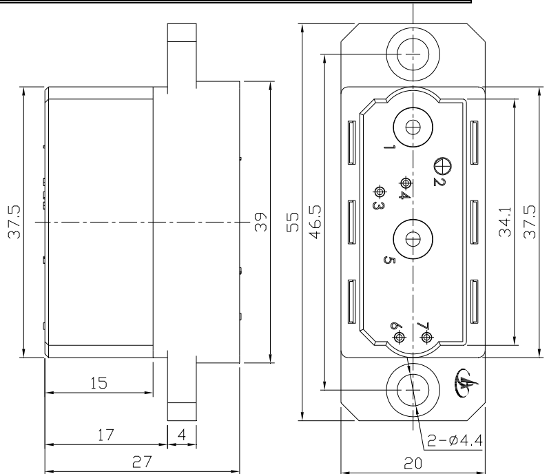
插头 JDS-07AZ
