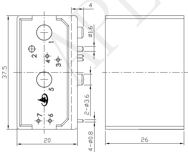
插座 JDS-07AT
