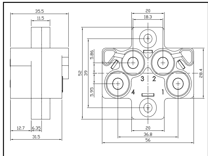
插头 JDS-04T
