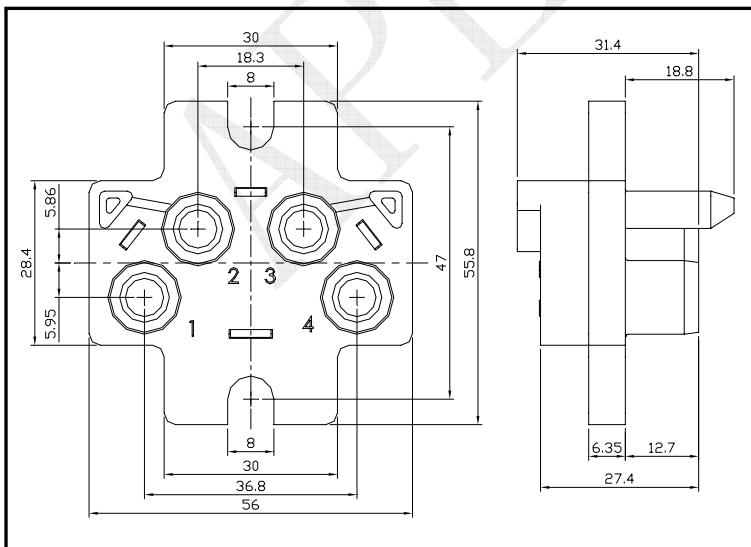
插座 JDS-04Z
