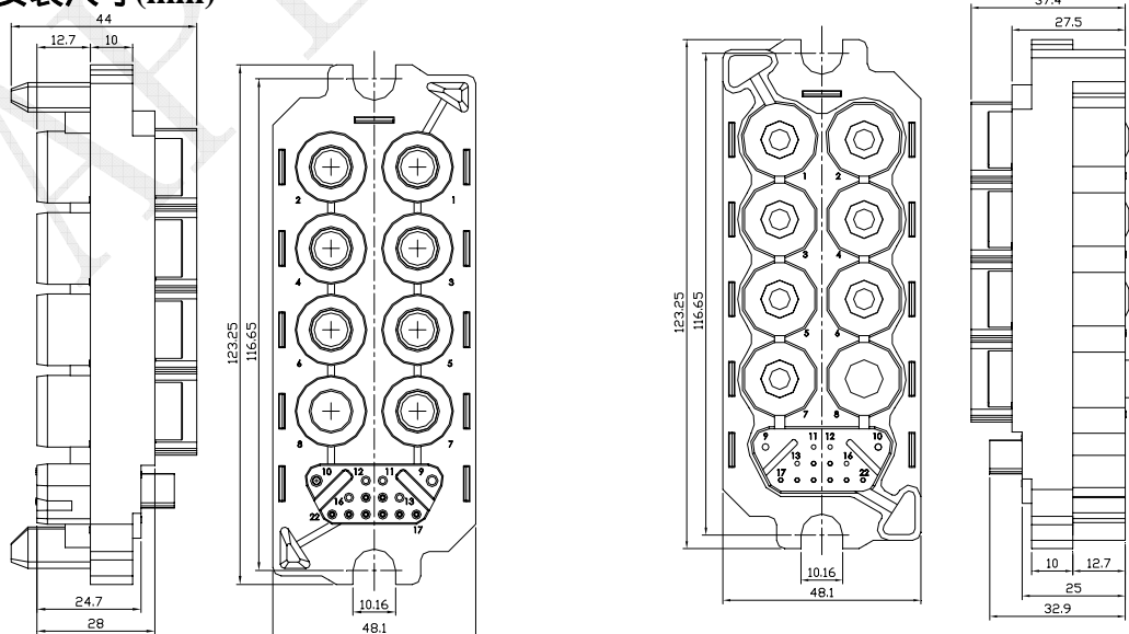
插座 JDS-22Z
