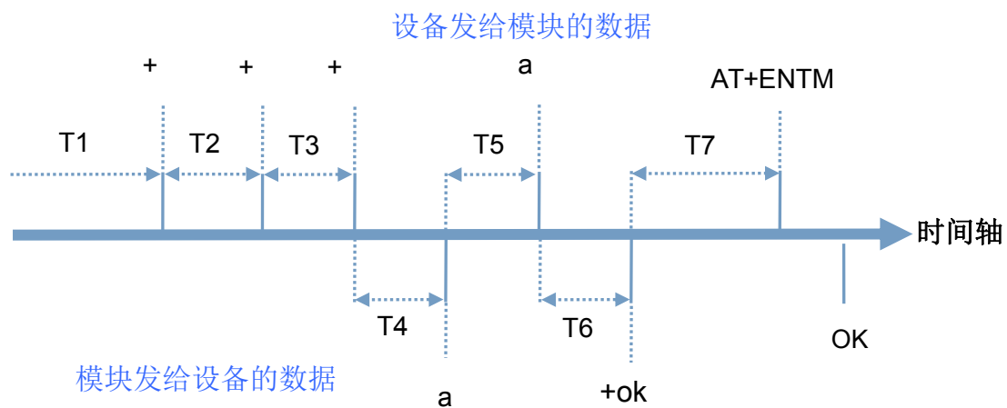
图 7 切换指令模式时序
