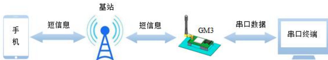
图 6 短信透传模式
