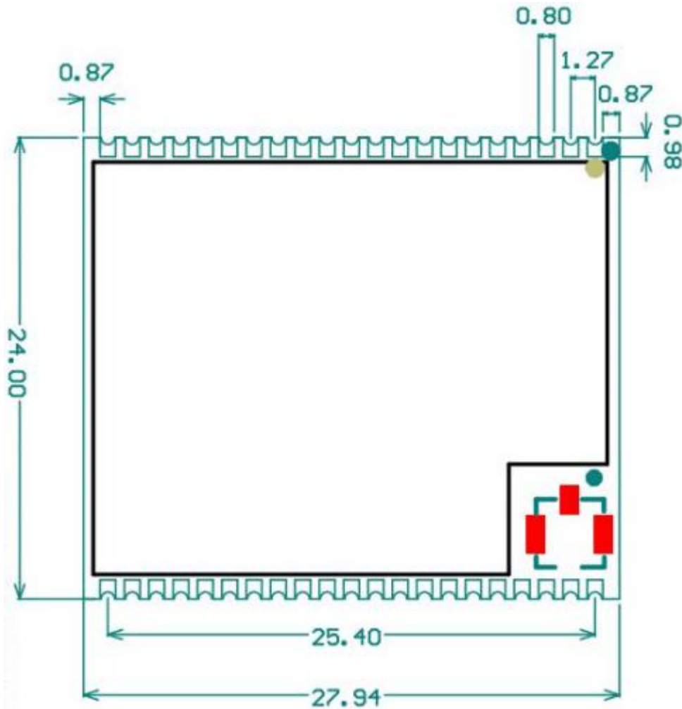
图 3 USR-GM3 尺寸图
