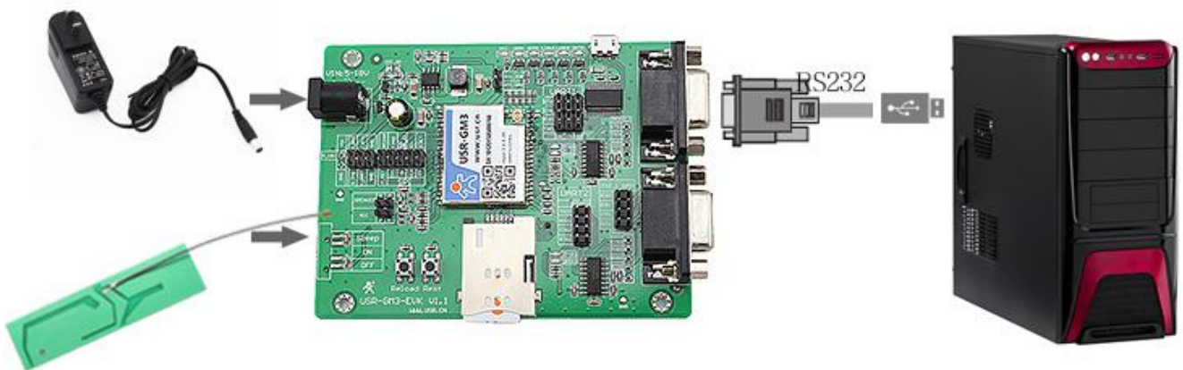
图 1 USR-GM3 硬件连接
