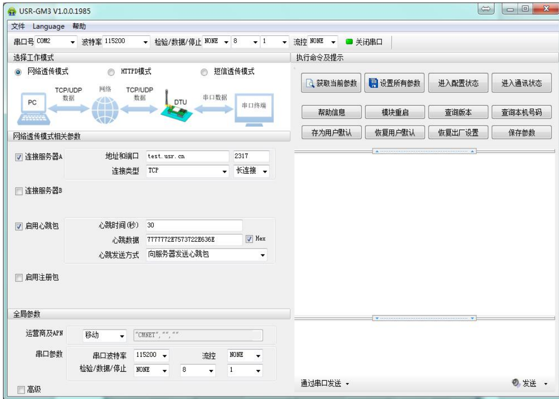
图 2 USR-GM3 设置软件
