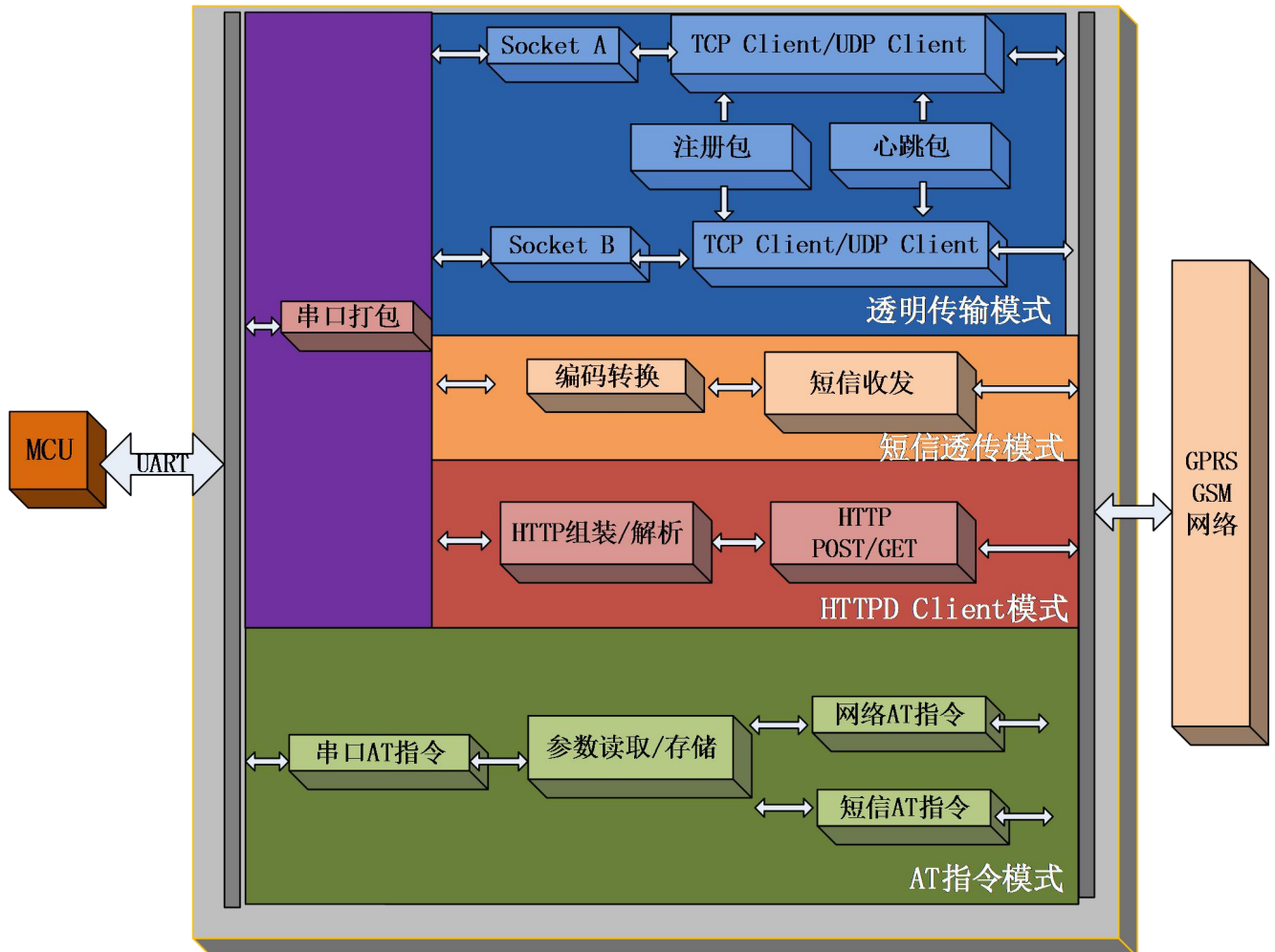
图 3 USR-GM3 功能框图
