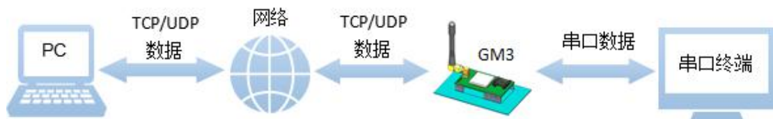
图 4 网络透传模式
