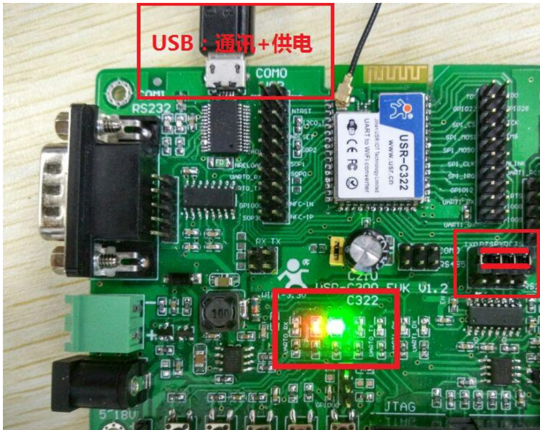
图 1 硬件连接图
