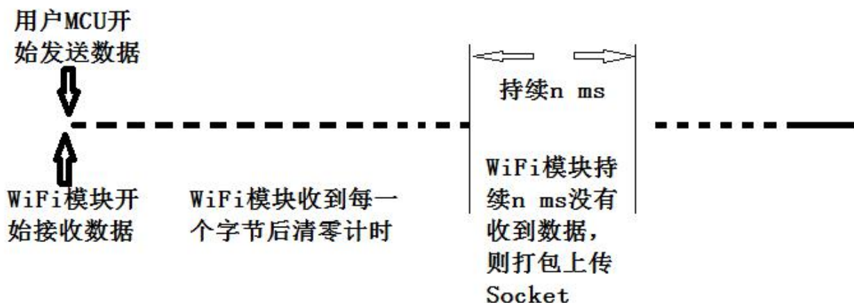
图 6 成帧机制
