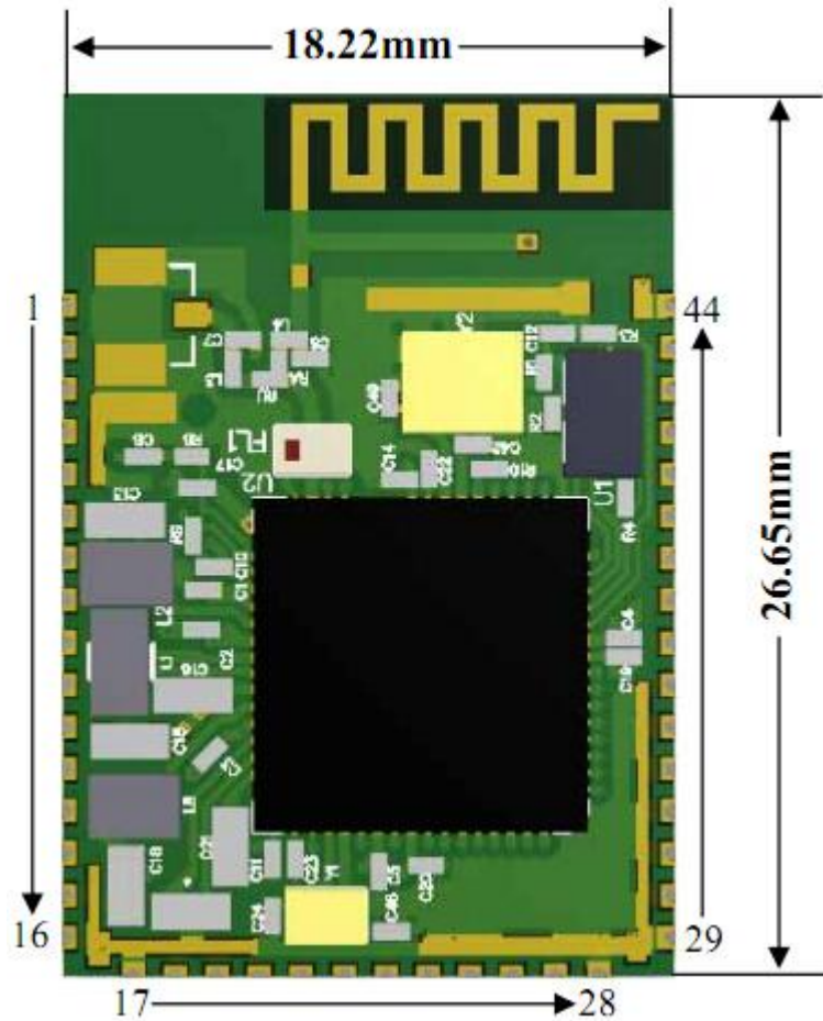
图 3 USR-C322 引脚图
