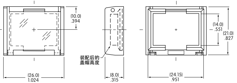
防护装置
