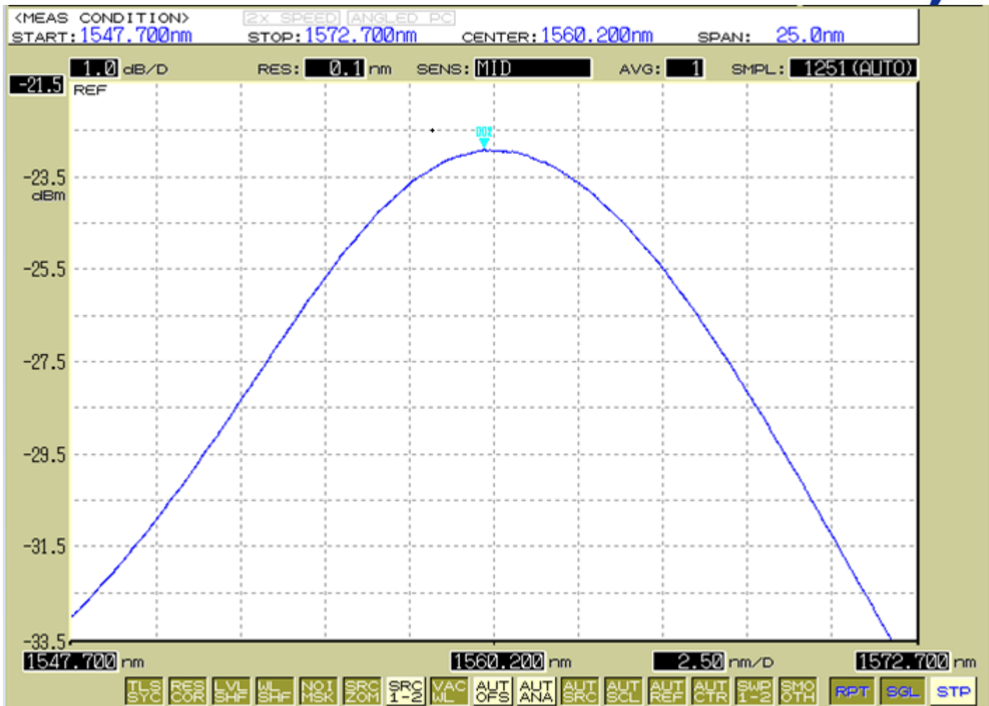
高斯型 ASE 光谱
