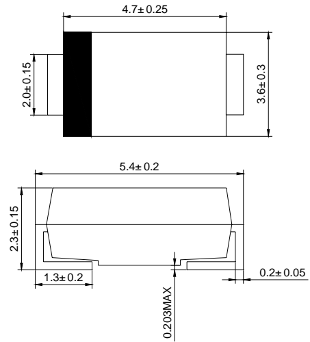
SMB (DO-214AA)
