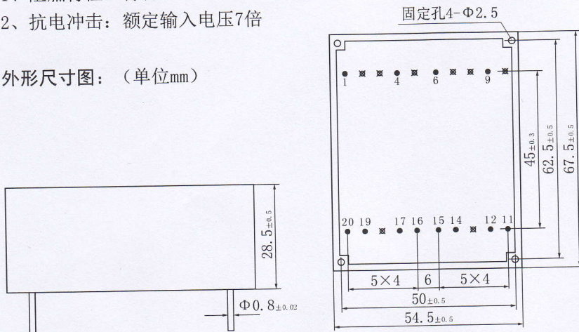
底视图（做PCB板时需注意）
