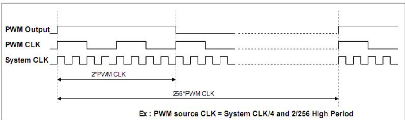
图 5-3 PWM 的 Duty
