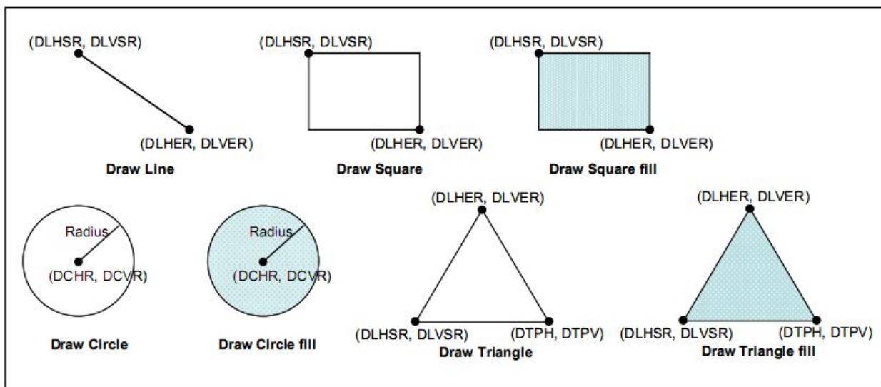
图 5-4 绘图功能参数
