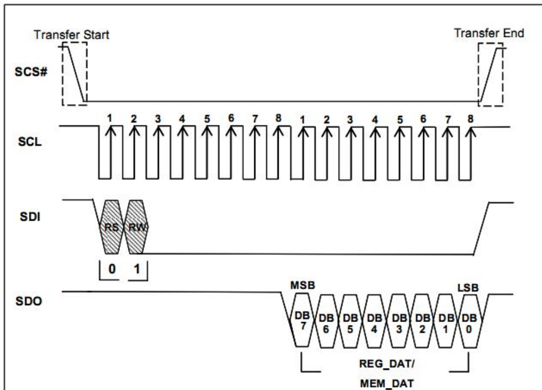
图 4-10 4-Wire SPI 数据总线的读取
