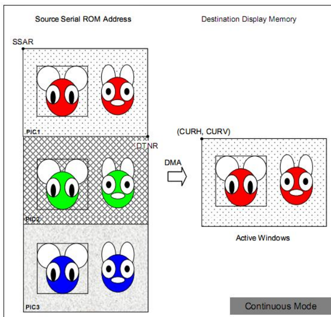
图 6-67 连续数据存储器存取模式
