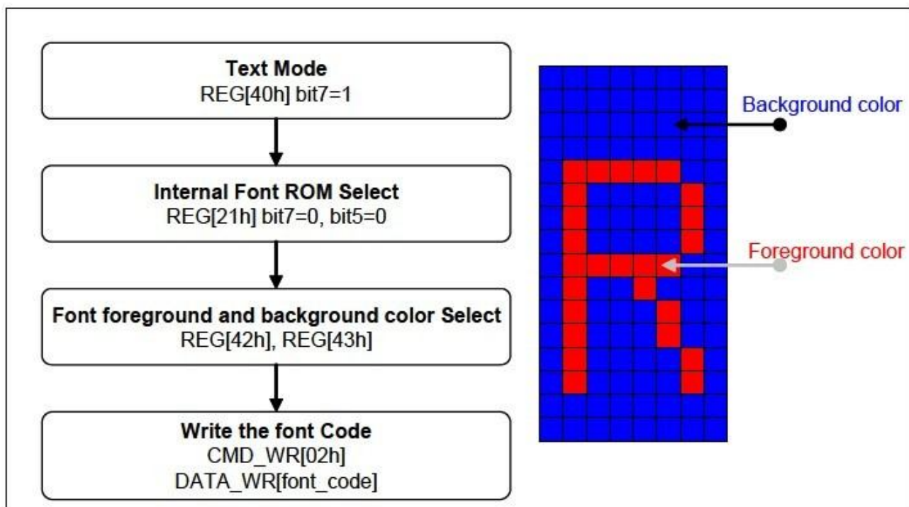
图 6-5 ASCII 字型 ROM 的写入程序
