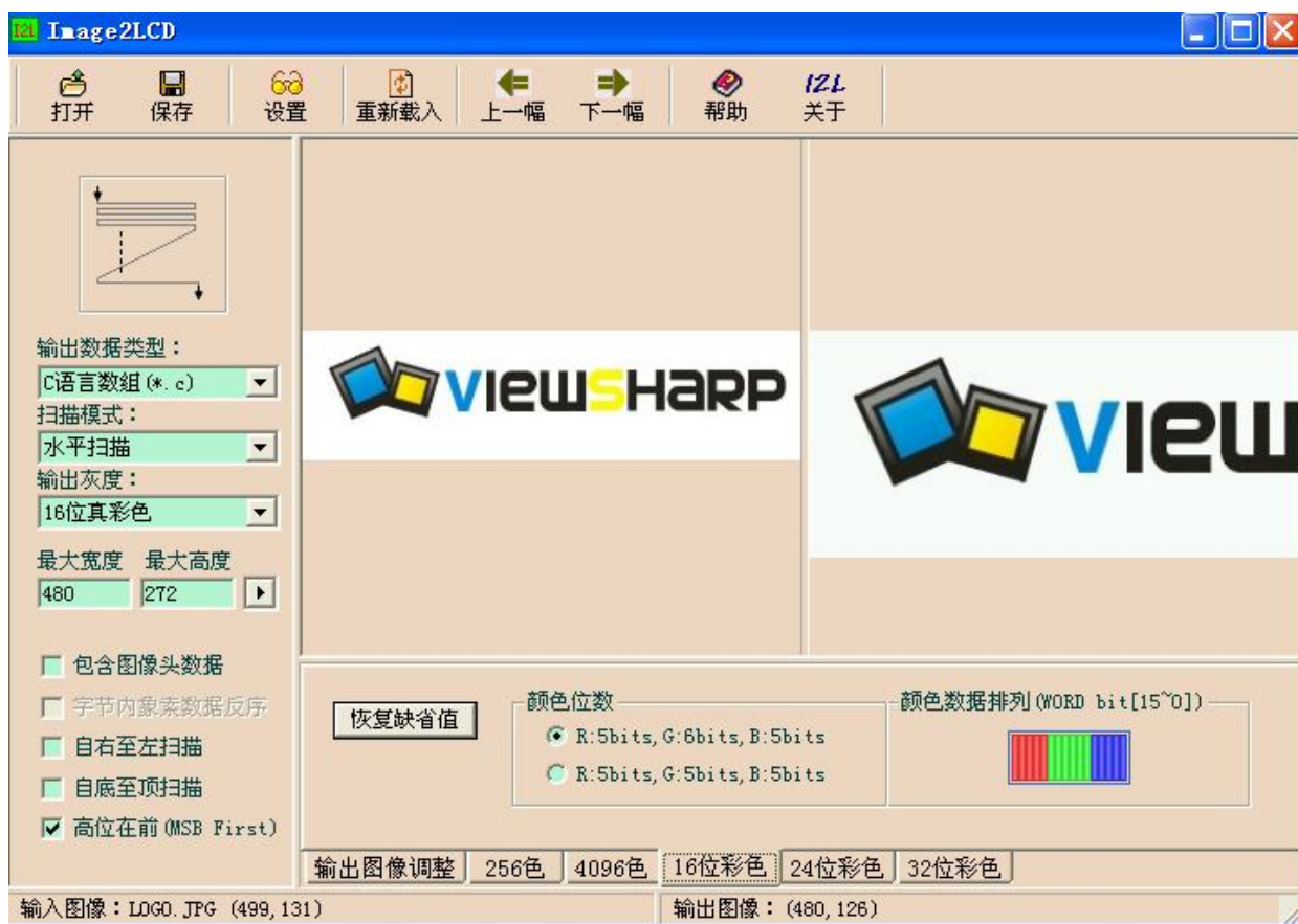
图 9-1 (彩屏取模软件应用界面)
