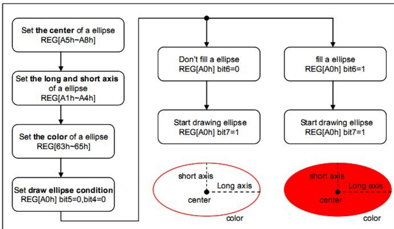
图 6-14 绘图功能 - 画椭圆
