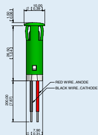
WIRES
