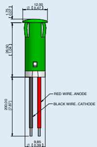
WIRES
