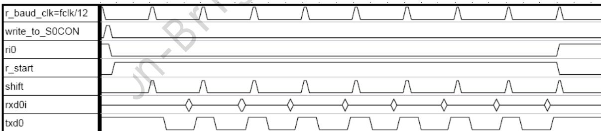
图 8-2: 接收模式 0
