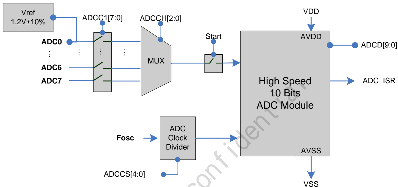
图 17-1: ADC 模拟到数字转换器的操作设置
