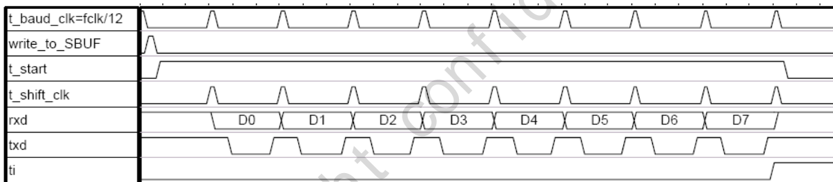
图 8-1: 发送模式 0
