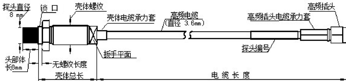
图 4 \phi 8 传感器探头示意图
