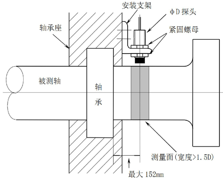
图 3.2 轴的径向振动测量时探头的安装
