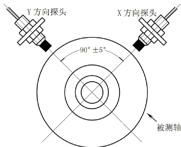
图 3.1 轴的径向振动测量
