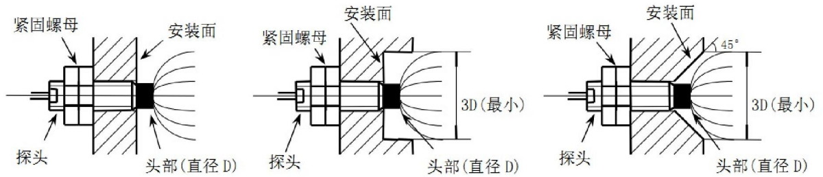
图 3.3 探头头部与安装面的距离图
