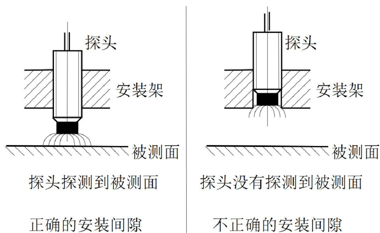
图 3.5 探头安装间隙正误图
