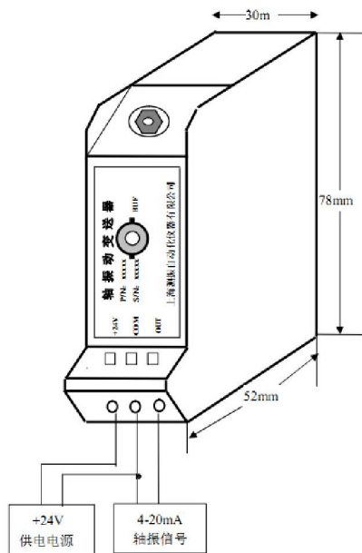
图 3.6 变送器连接
