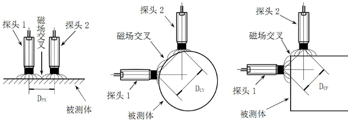
图 3.4 各探头间的距离图
