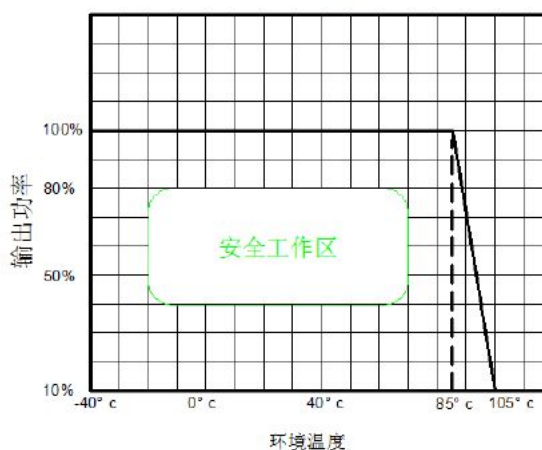
温度曲线图
