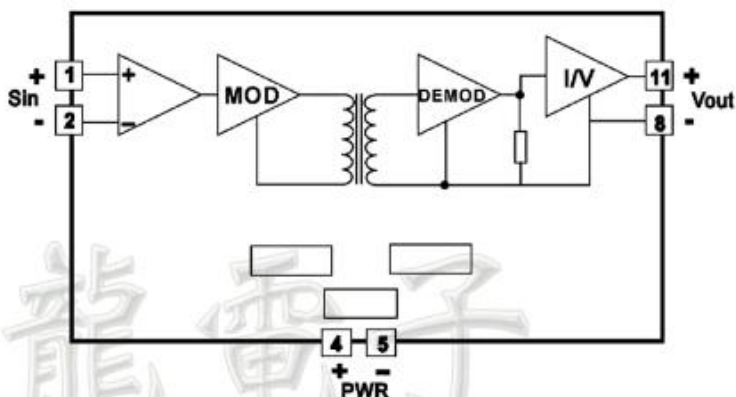
简易连接图
