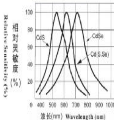
光谱响应特性 Spectral Response
