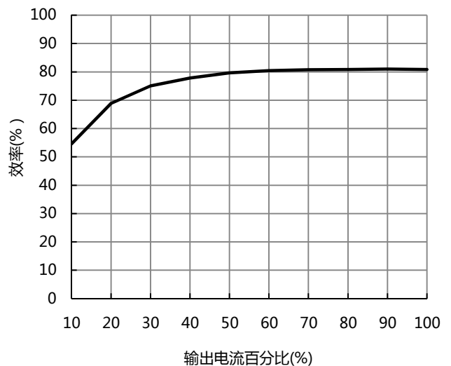
图 6. B0505S-1WR2 效率 vs 输出负载 (标称输入)
