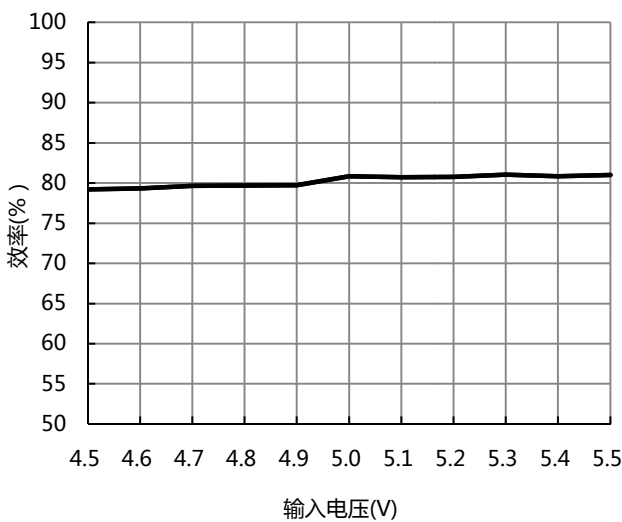
图 5. B0505S-1WR2 效率 vs 输入电压 (满载)
