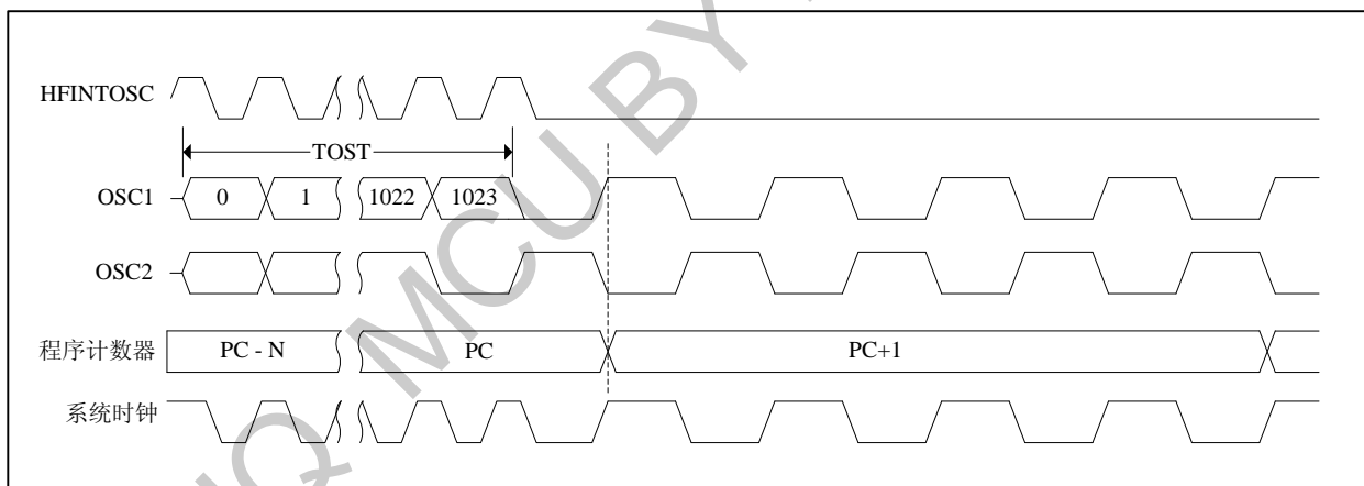
图 4-7-3: 双速启动
