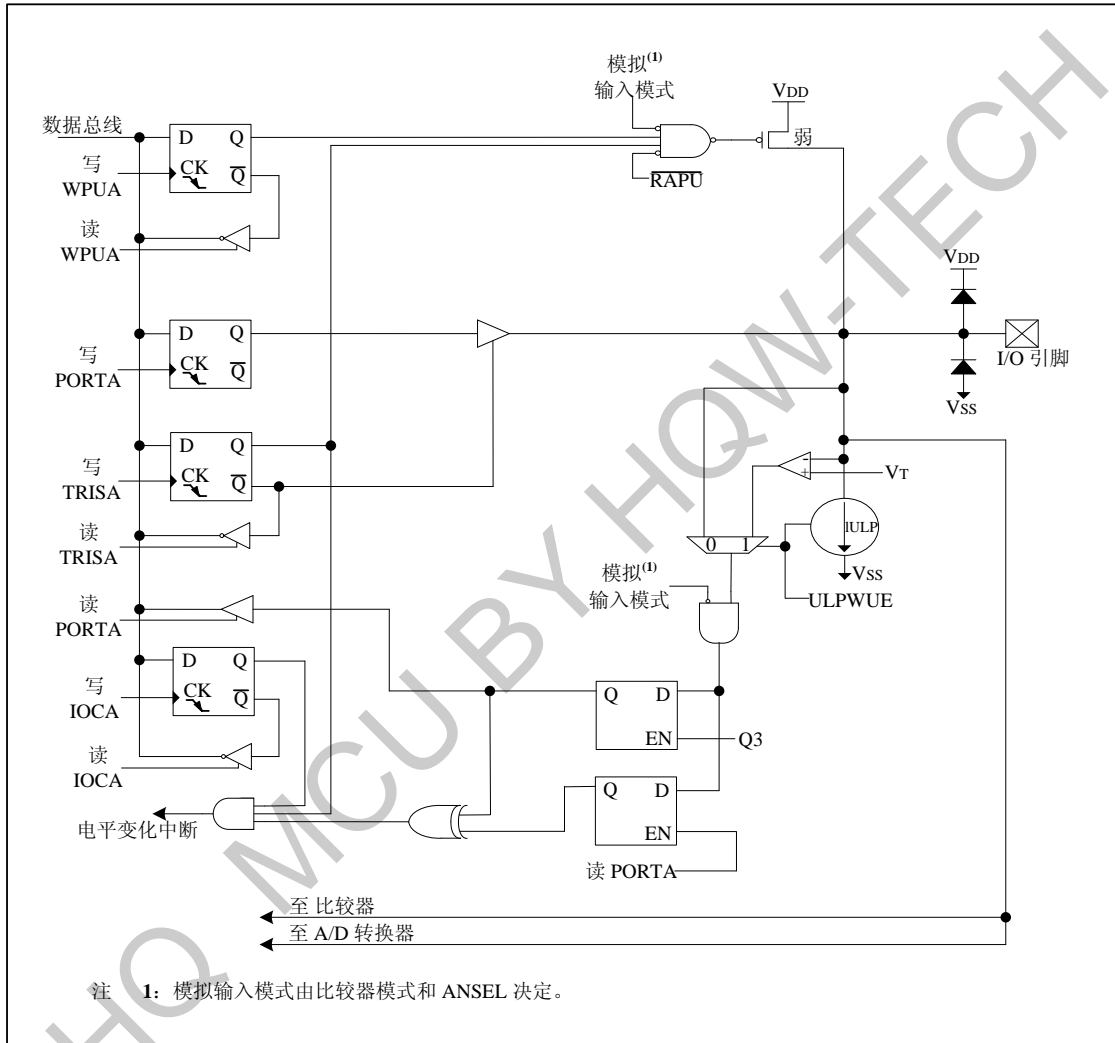
图 6-4-1: PA0 框图
