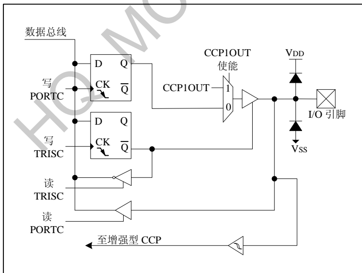
图 6-5-6: PC5 框图
