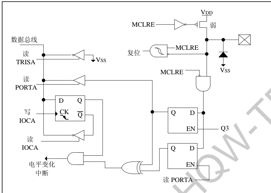
图 6-4-4: PA3 框图
