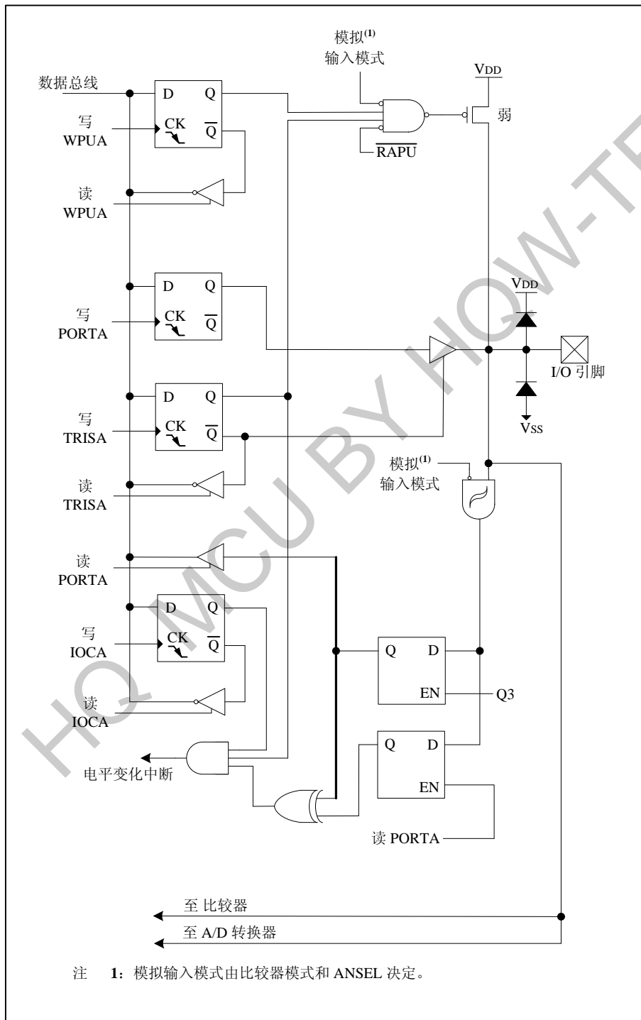
图 6-4-2: PA1 框图
