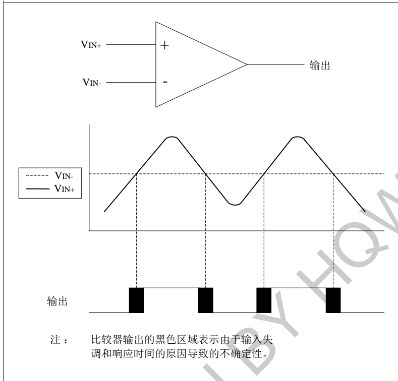
图 10-1-1: 单比较器
