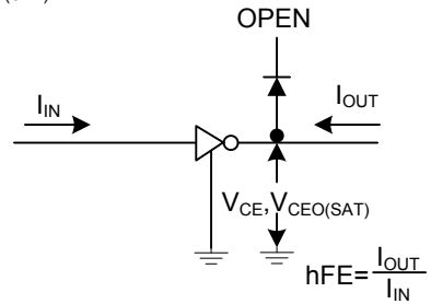
2. V_{CEO(SAT)}, h_{FE}
