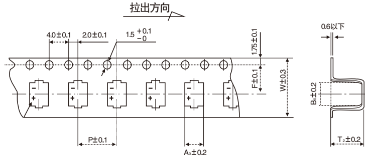
Fig.1 (适用于Φ10以下产品)
