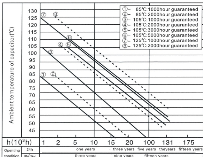
(图2-1 寿命推算曲线)
