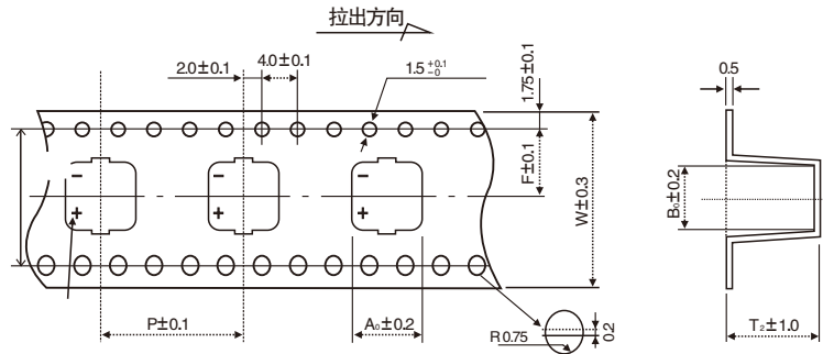
Fig. 2 (适用于Φ12以上产品)
