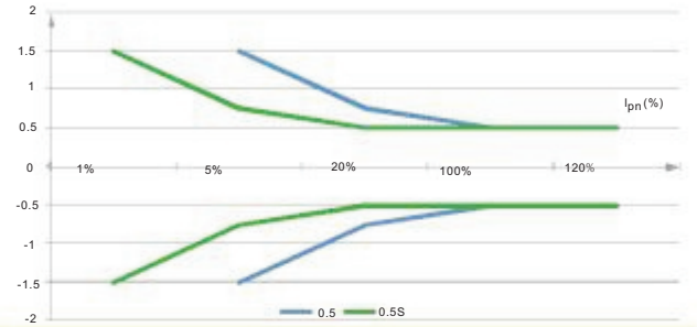
b) 精度0.5和0.5S的对比
