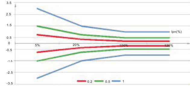
a) 精度类别: 0.2: 0.5: 1
