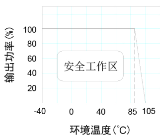
温度曲线图
