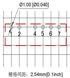
推荐 PCB 图
