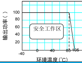
温度曲线图
