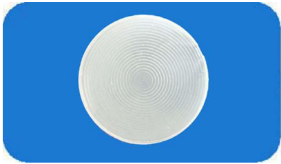
型号: 8250(平板形) 焦距: 25 角度: 30° 距离: 10m 尺寸: Ø13 厚度:0.5
