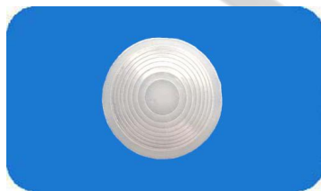
型号: 8180(平板形) 焦距: 20 角度: 30° 距离比:6:1 尺寸: Ø18
