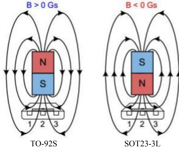
单极开关型
