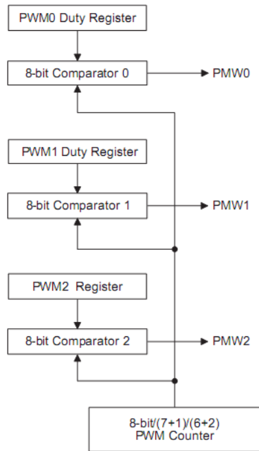
PWM 方块图
