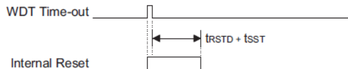
正常运行时看门狗溢出时序图
