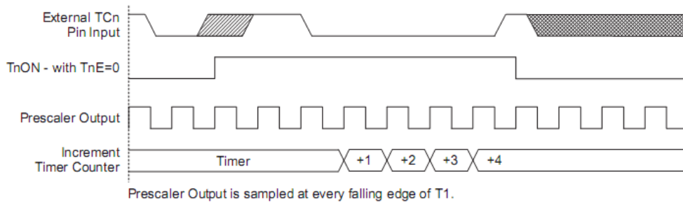
脉冲宽度测量模式时序图 (TnEG=0)
