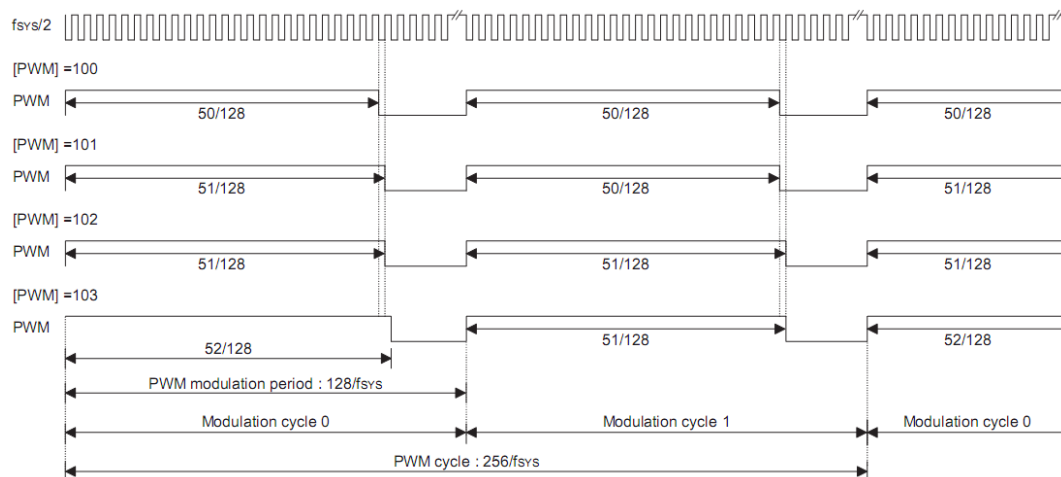
7+1 PWM 模式
