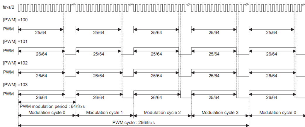
6+2 PWM 模式
