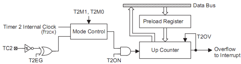
8 位定时/计数器 2 结构图
