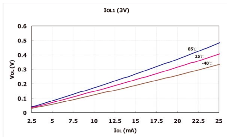
V OL 与 I OL1 之间的过温关系图 (V DD =3.0V)
