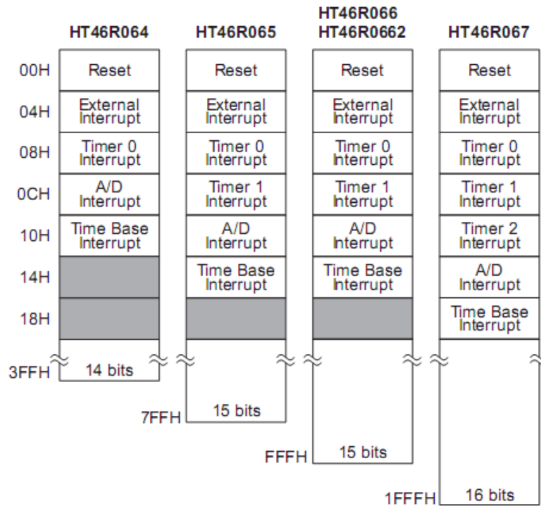
程序存储器结构
