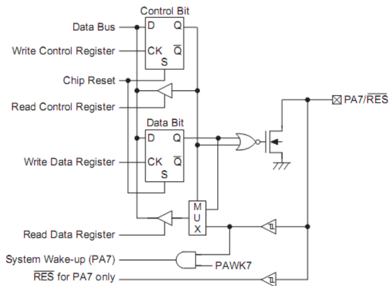
PA7 NMOS 输入/输出端口
