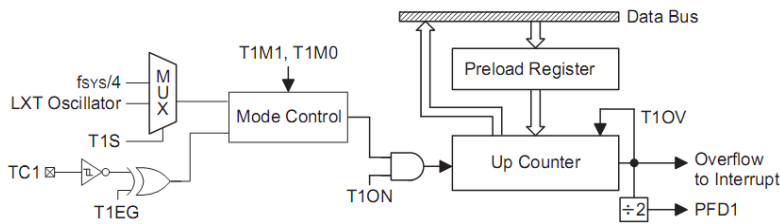
8 位定时/计数器 1 结构图
