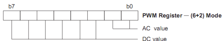
6+2 模式时的 PWM 寄存器
