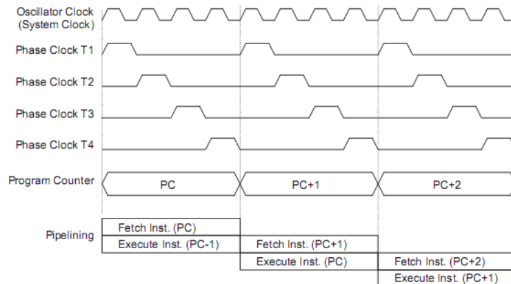
系统时序和流水线
