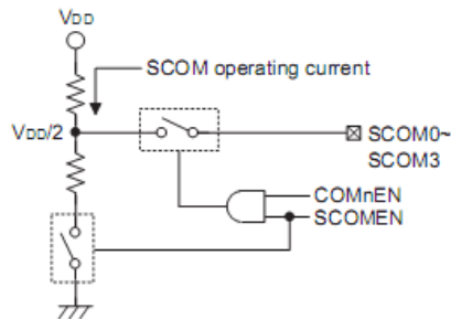
SCOM 电路
