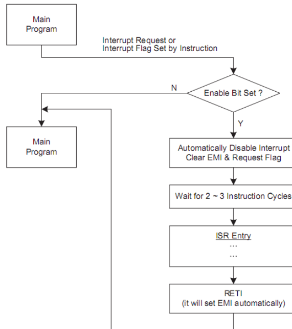
中断流程图
