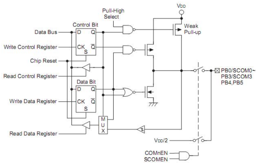
PB 输入/输出端口
