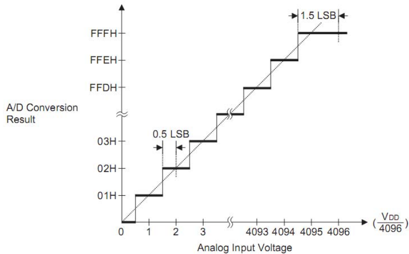
理想的 A/D 转换功能
