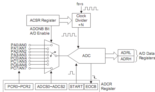
A/D 转换器结构
