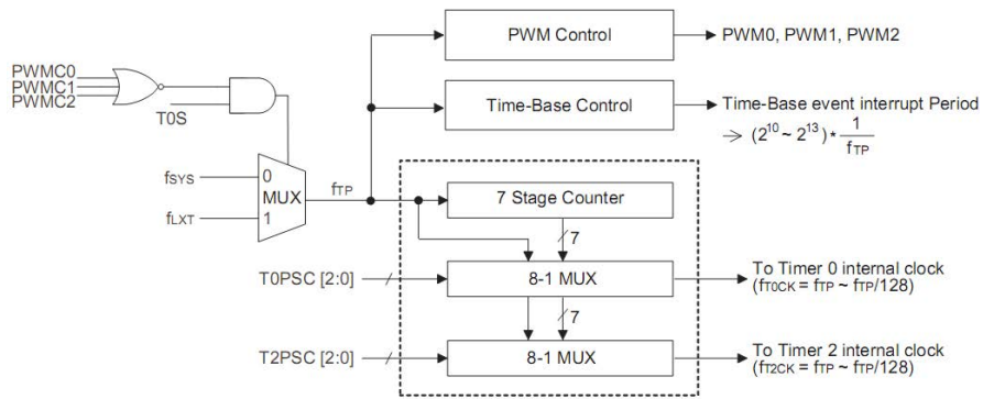
Timer/PWM/Time Base 的时钟源结构图
