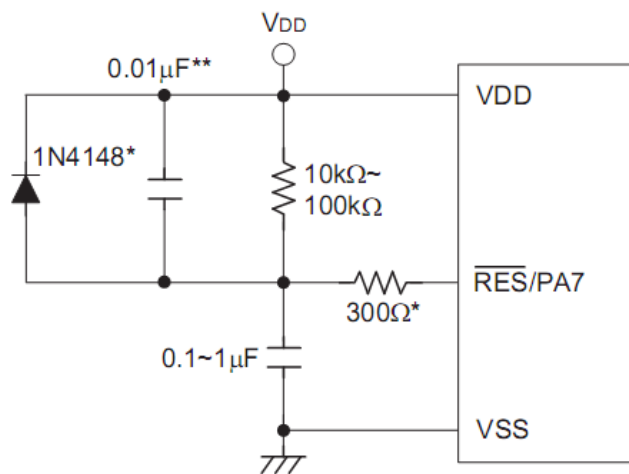
外部RES电路
