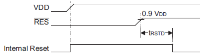
上电复位时序图
