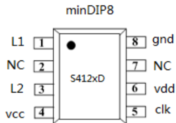
图2 脚位图
