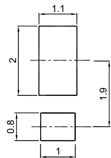
SOD-323HE
