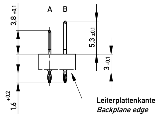
Kontaktversionen, Messerkontakte Contact Selection Options, Male Contacts
