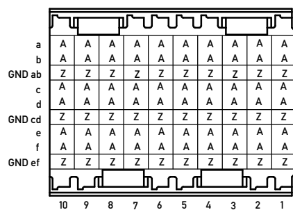
Bestückungsplan - contact layout
