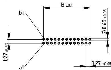
Layout M 2:1
