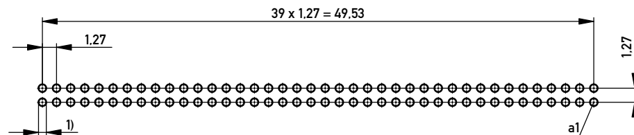
Lochbild für Leiterplatte Board hole pattern
