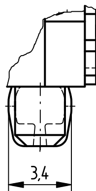
Ansicht X M 5:1
