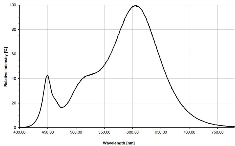
F2 Spectral:
