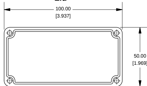
Lid
