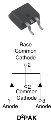
16CTU04SPbF
