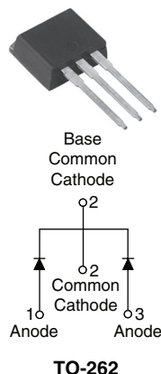
16CTU04-1PbF
