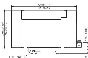
VIEW A.
