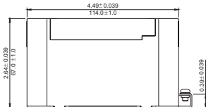
VIEW A.
