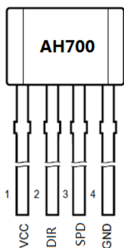
TO94
