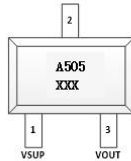
SOT23-3L
