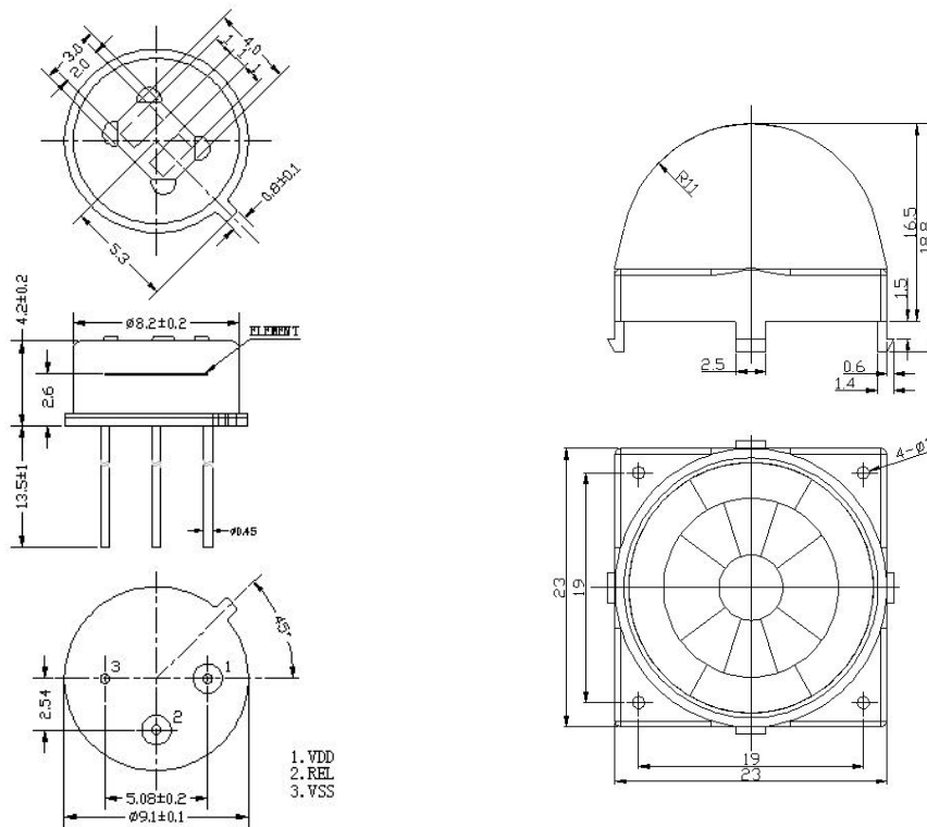
探头外观图 (A)
