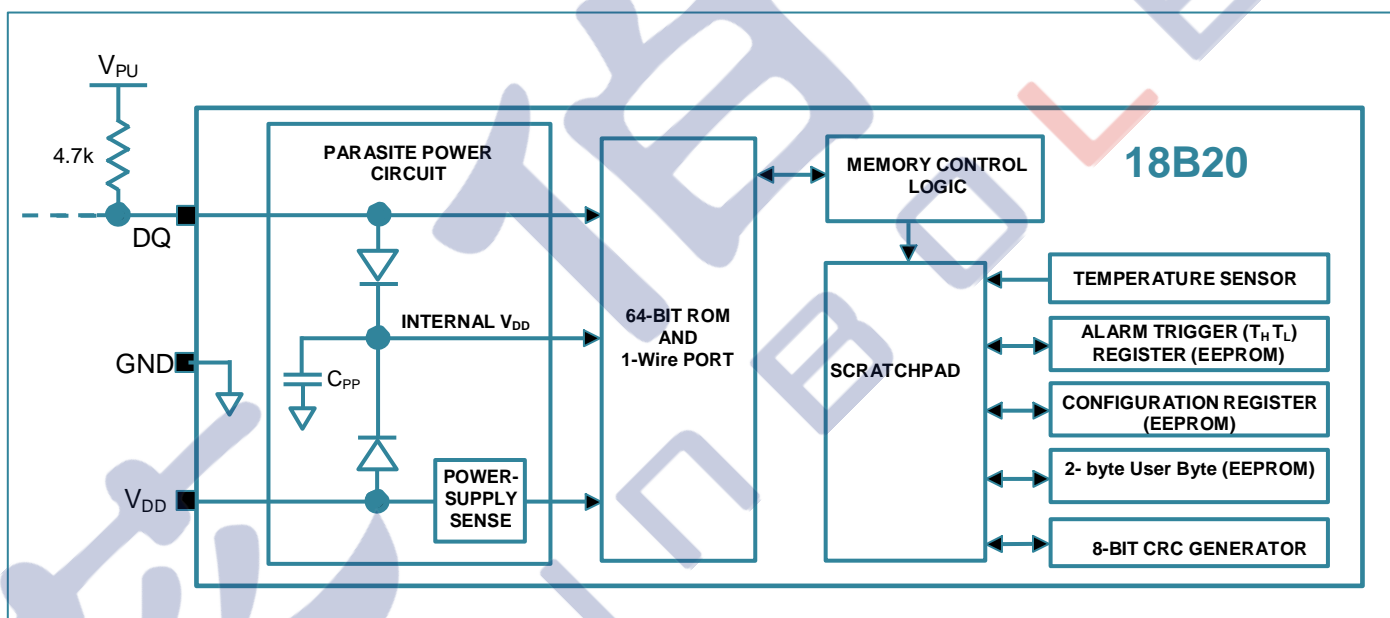
图 1. 18B20 的结构框图
