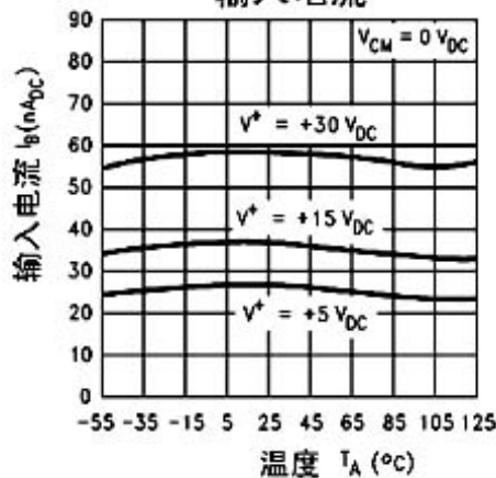
输入电流
