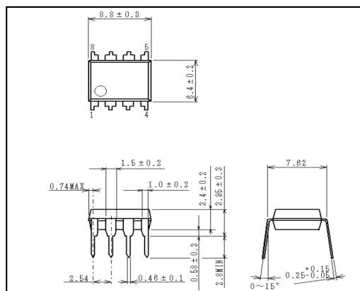
封装外形图
