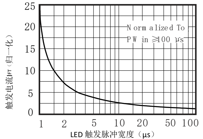
图4 触发电流 vs LED 脉冲宽度
