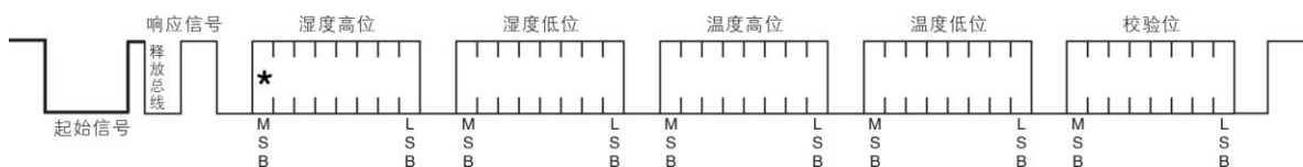
图 5： AM2301 单总线通信协议
