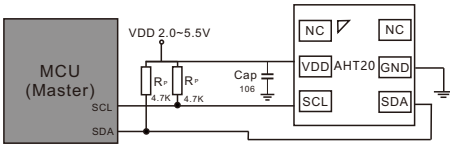
图16 典型应用电路
