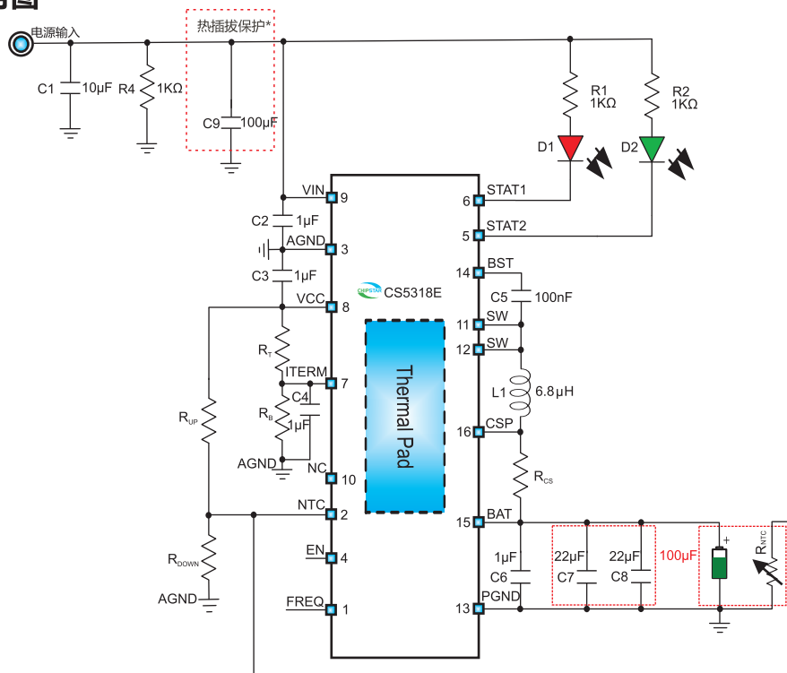
CS5318E应用电路图
