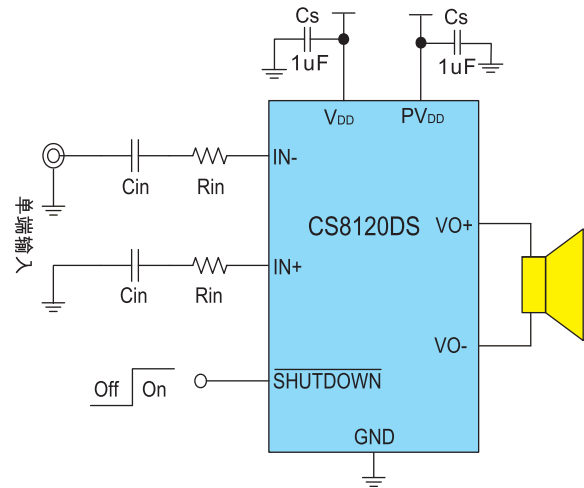
图2 CS8120DS单端输入方式应用图
