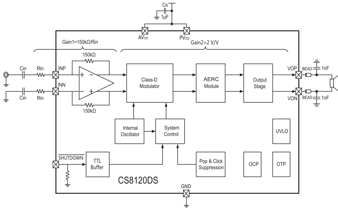
CS8120DS功能框图
