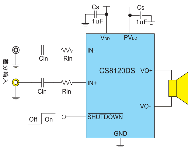
图1 CS8120DS差分输入方式应用图
