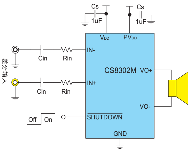
图1 CS8302差分输入方式应用图
