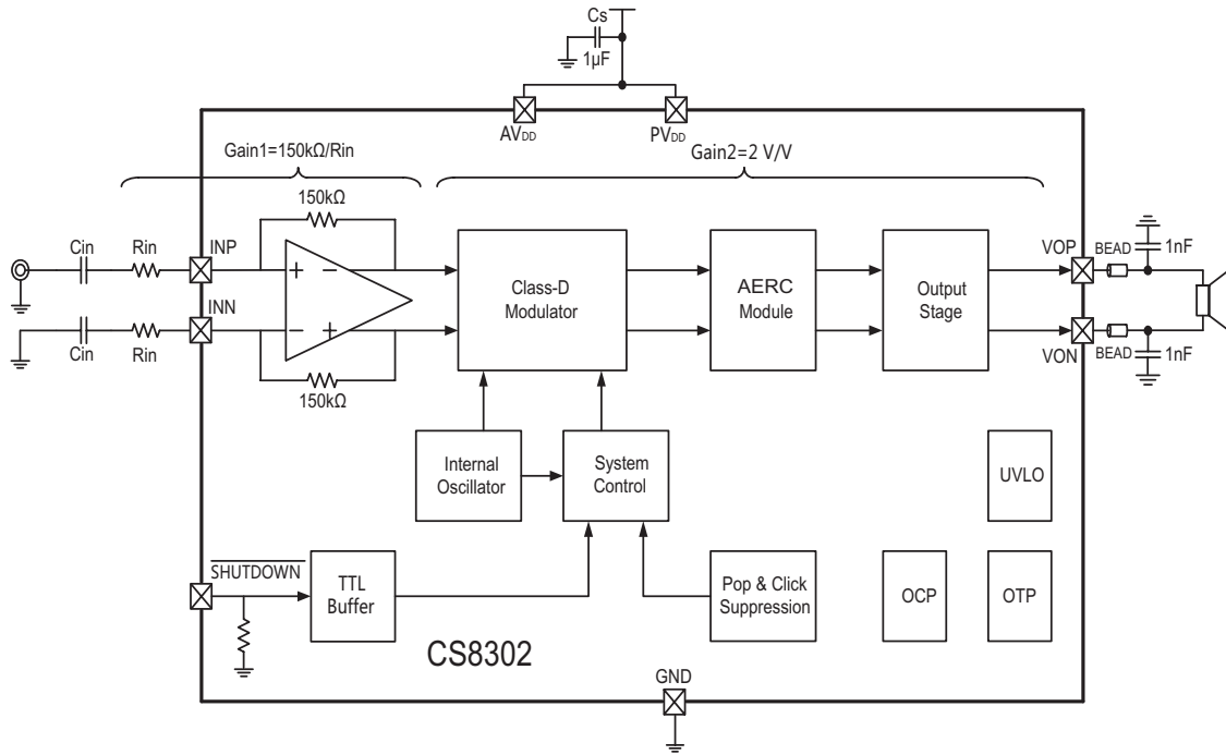
CS8302功能框图
