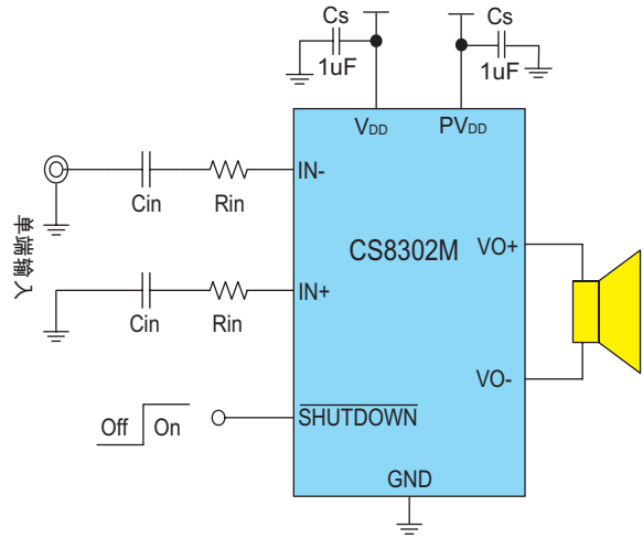
图2 CS8302单端输入方式应用图
